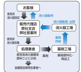
●消火器のリサイクルシステム
