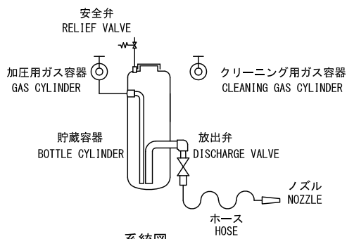
系統図 SYSTEM DIAGRAM
