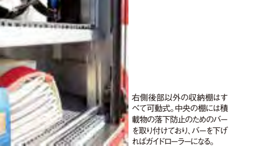
右側後部以外の収納棚はすべて可動式。中央の棚には積載物の落下防止のためのバーを取り付けており、バーを下げればガイドローラーになる。
