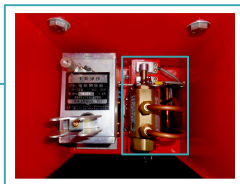
起動操作管閉止弁 HB-K-01
