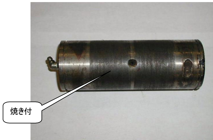
写真2 軸受部(根本ピン)
