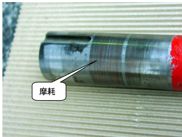
写真10 梯体起伏軸
