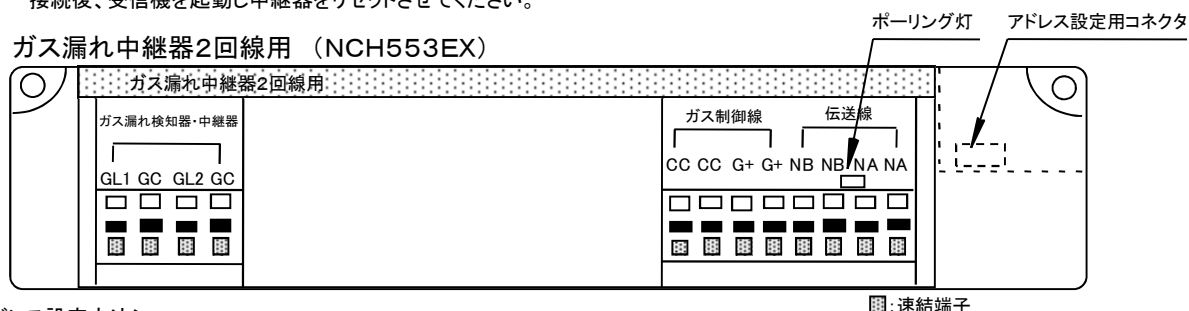
図: 連結端子
