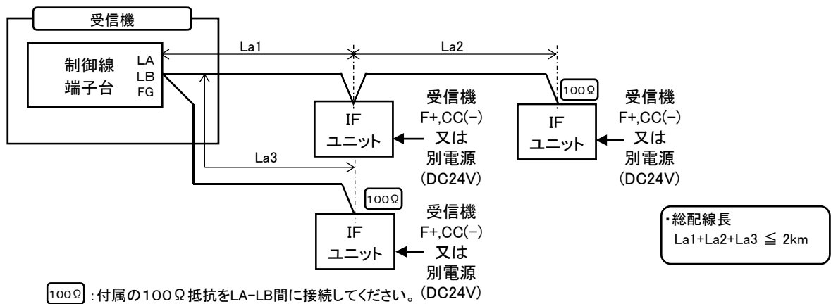
<b:バス型 2>
