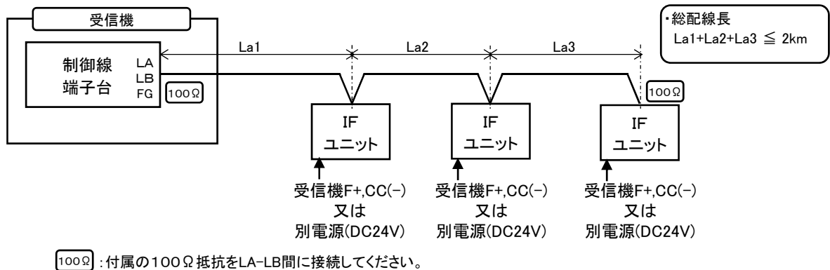
<a:バス型 1>
