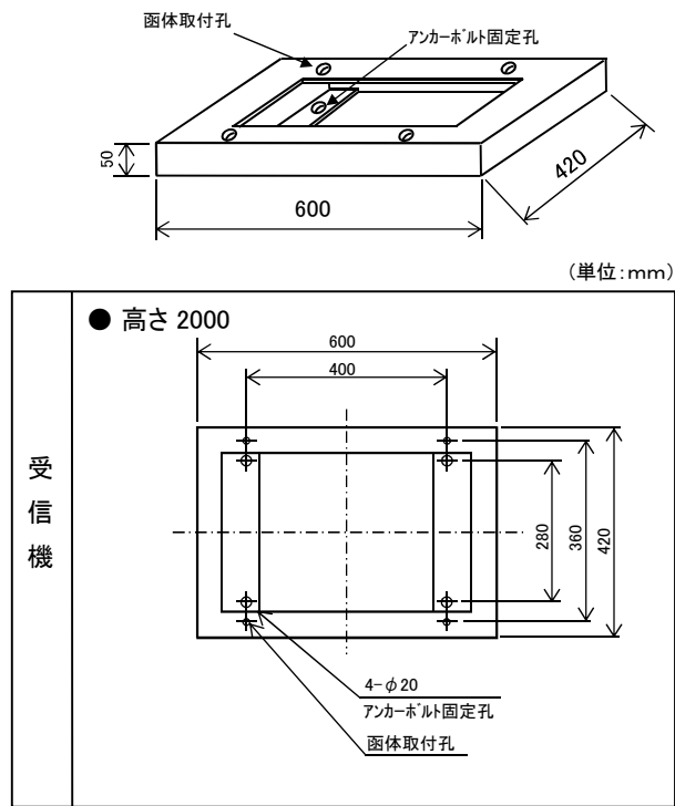
【図2】受信機チャンネルベース寸法図 標準寸法図(単位:mm)
