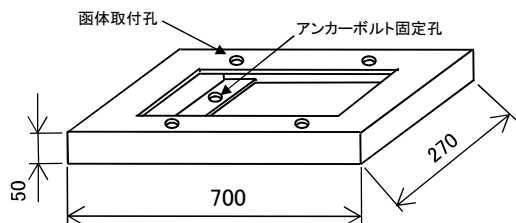
【図5】分散処理盤チャンネルベース寸法図 標準寸法図(単位:mm)
