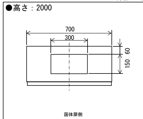
【図6】分散処理盤函体の入線孔寸法図 入線孔は筐体上面と底面にあります。
