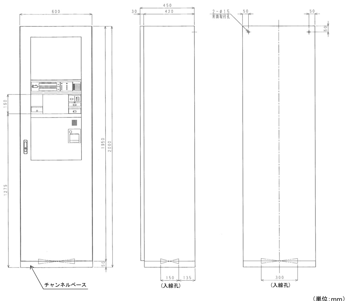
【図1】取付寸法図 (H2000×W600×D450)
