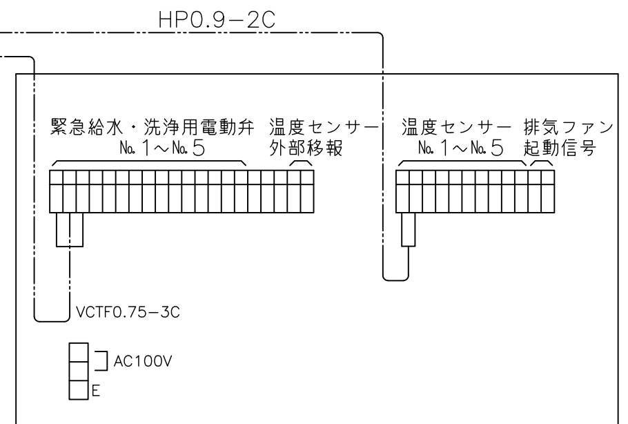
制御盤内部配線図
