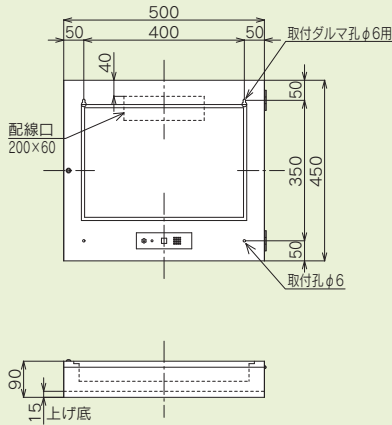
地図式副受信機埋込型内器 NYI407FK
