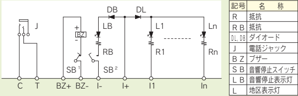
副受信機内部回路図 地図式副受信機 NYI407
