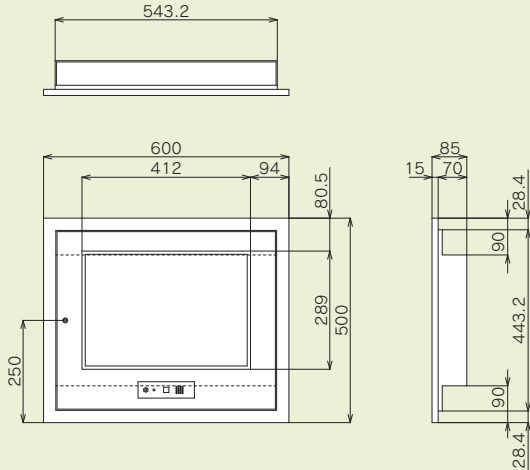
地図式副受信機埋込型内器 NYI407FK
