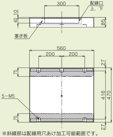
埋込ボックス NBY422FJ
