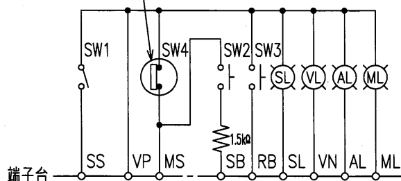
扉開時にSW4導通
