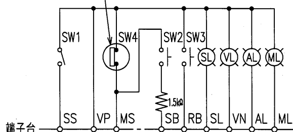
扉開時にSW4導通
