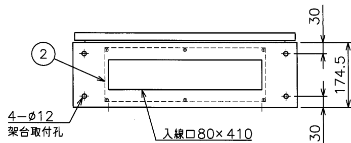
【盤取付孔（上部）詳細】
