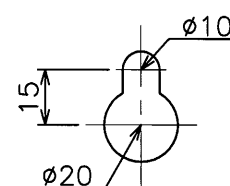
【盤取付孔 (上部) 詳細】
