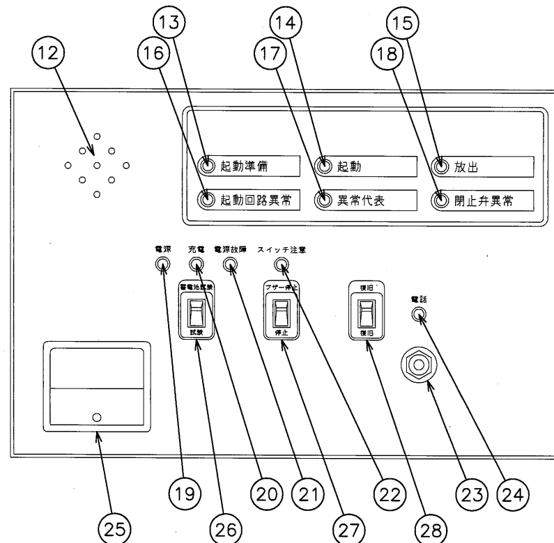
【B部詳細】
