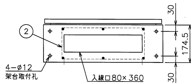
【盤取付孔（上部）詳細】
