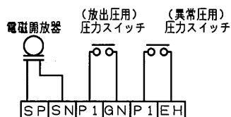
配線図 (極性なし)
