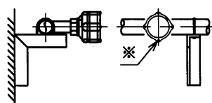
銘板詳細
