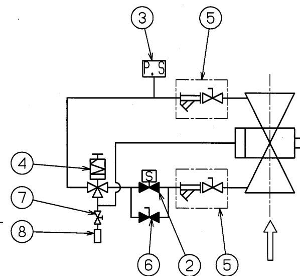
制御配管系統図
