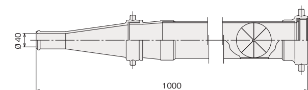
遠隔操作モニター用水ノズル
