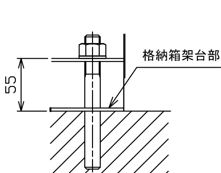
アンカーボルト取付状態例
