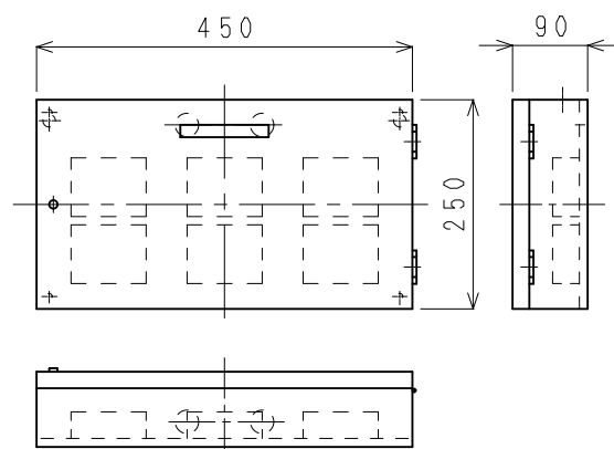
[RX] 熱電対式（自動試験対応）取付図
