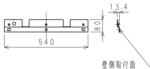
取付金具 (S=1/15)
