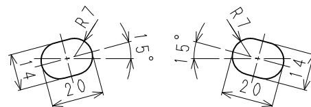
取付用長穴寸法図 (S=1/2)
