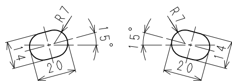
取付用長穴寸法図 (S=1/2)
