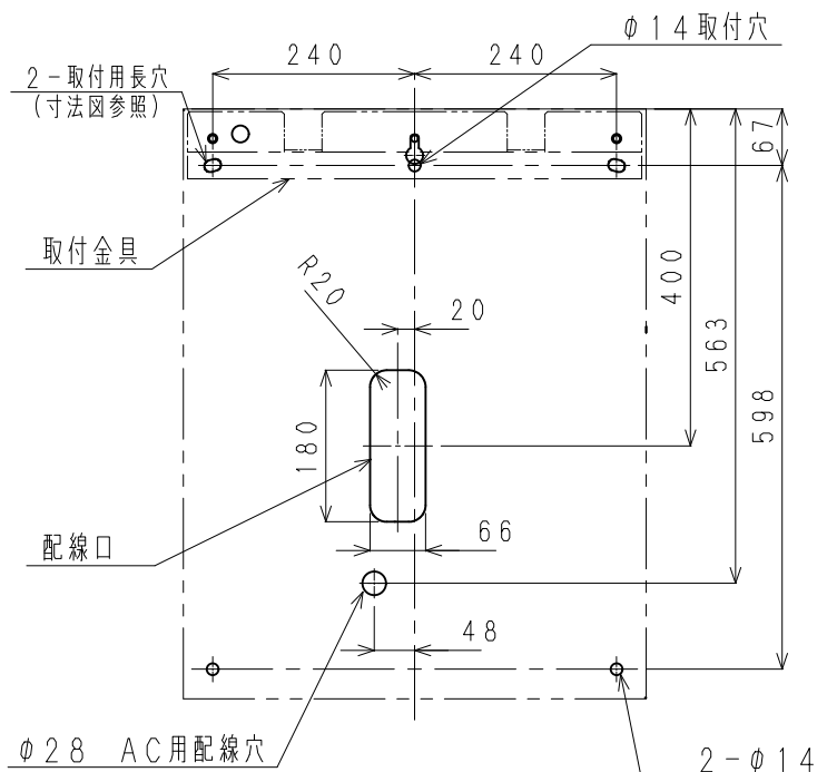
取付寸法図 (正面より)
