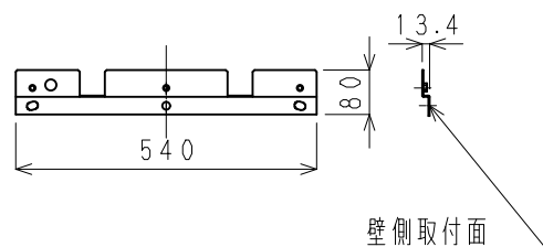
取付金具 (S=1/15)
