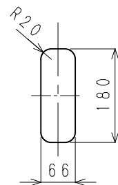
配線口寸法図 (S=1/10)
