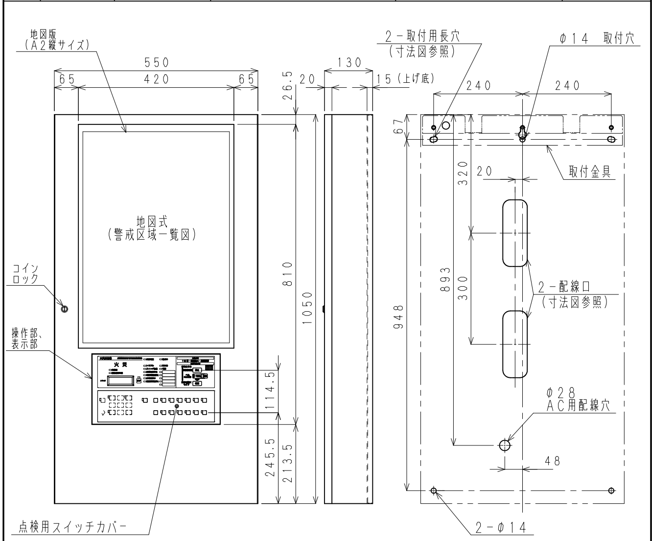
取付寸法図 (正面より)
