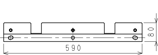
取付金具 (S = 1 / 10)
