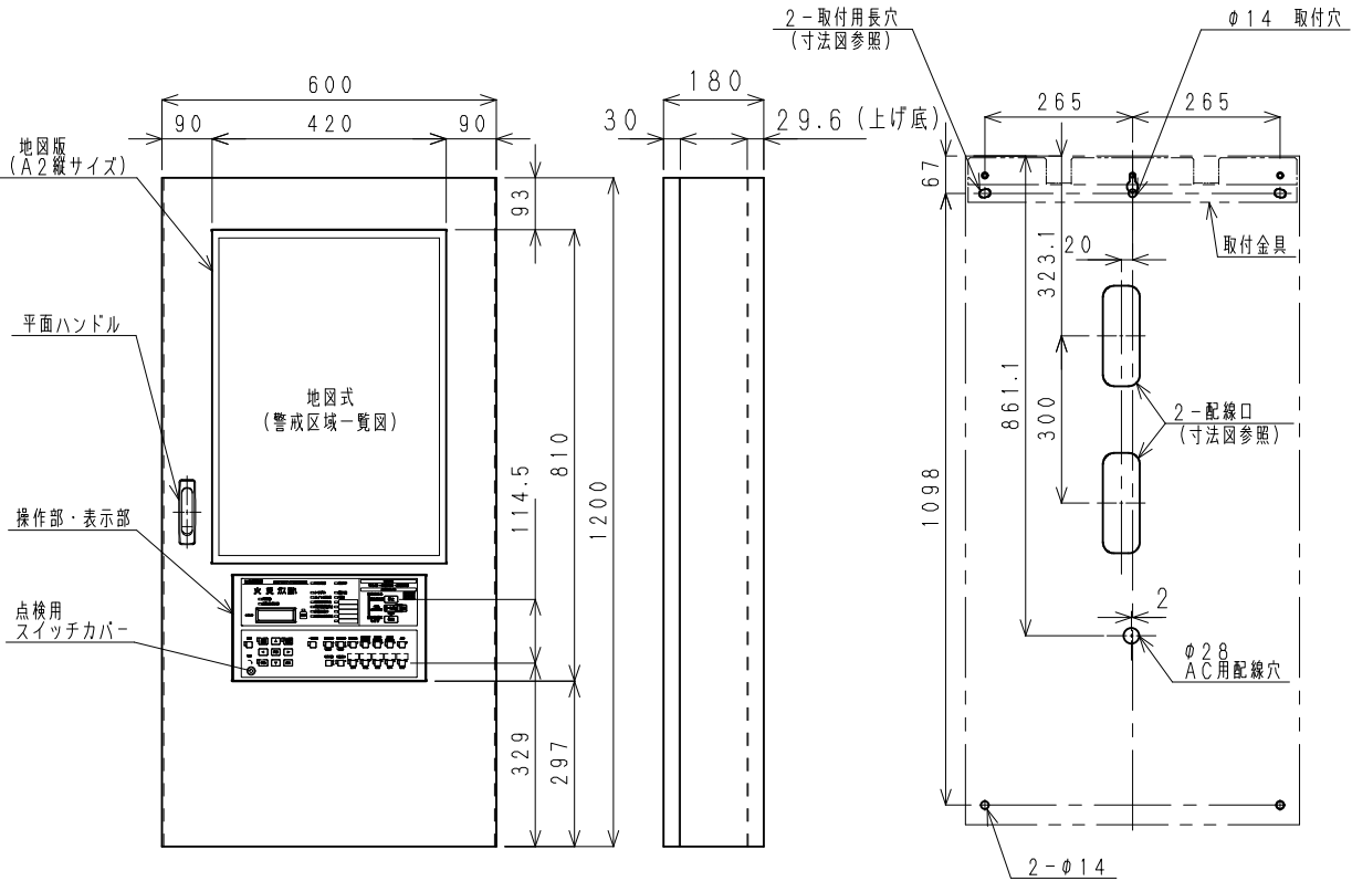
取付寸法図 (正面より)
