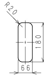
配線口寸法図 (S = 1 / 10)
