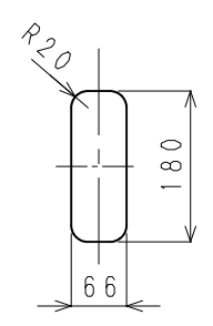
配線口寸法図 (S = 1 / 10)
