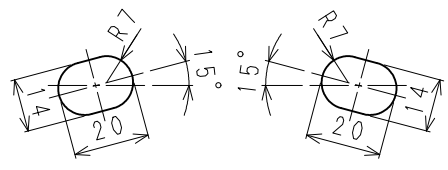
取付用長穴寸法図 (S = 1 / 2)
