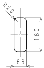
配線口寸法図 (S = 1 / 10)
