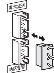
非常放送/地区音響切替コネクタ
