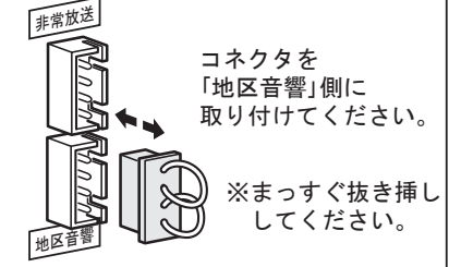
非常放送／地区音響切替コネクタ
