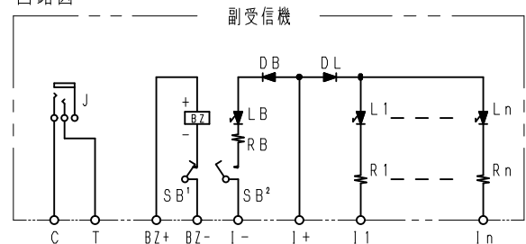
回路図
