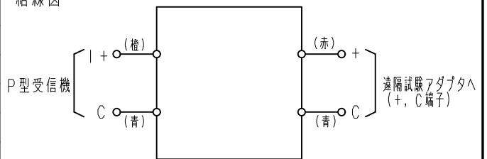
結線図
