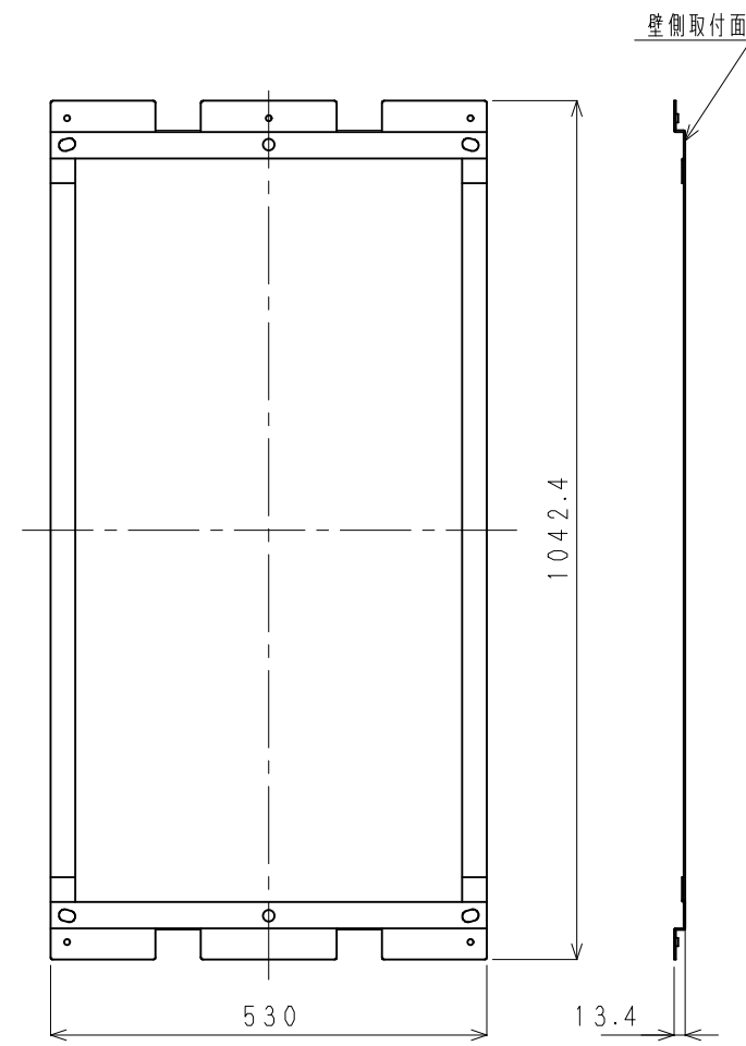
取付金具 (t = 2.0 : 防錆塗装)
