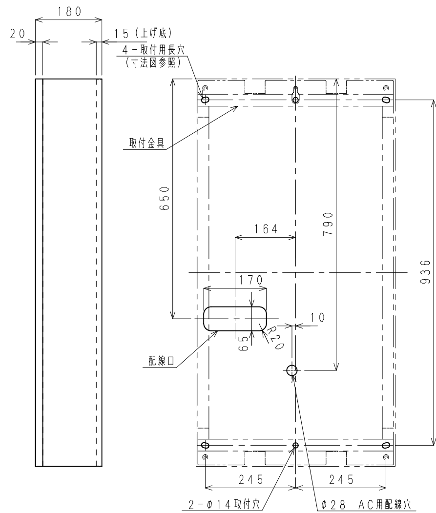
取付寸法図（正面より）
