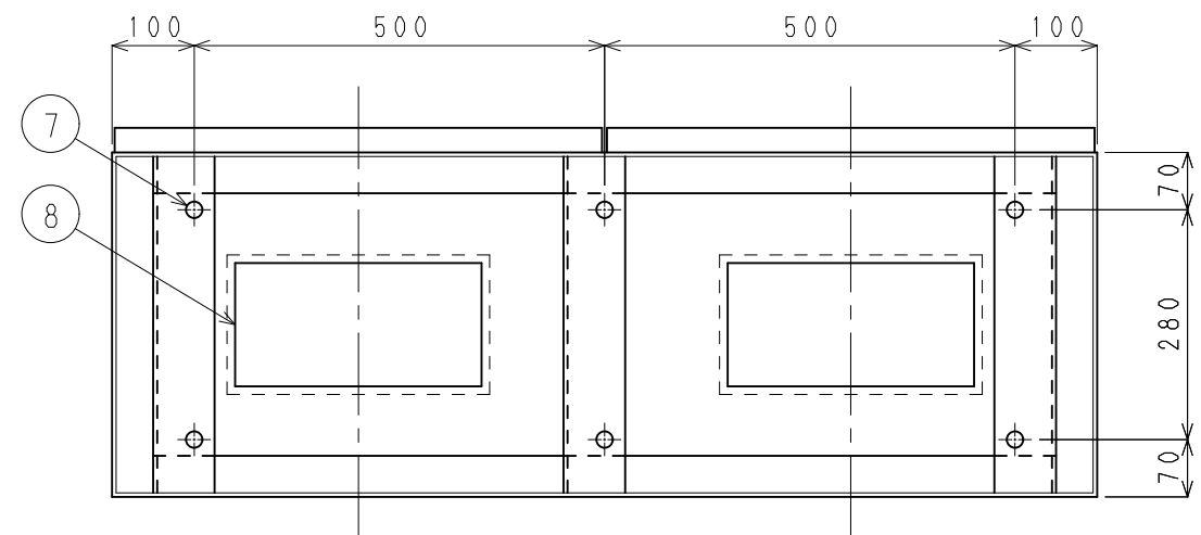
底面図
