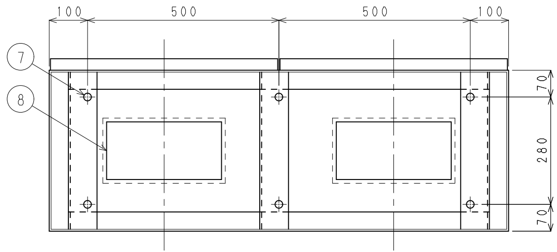
底面図
