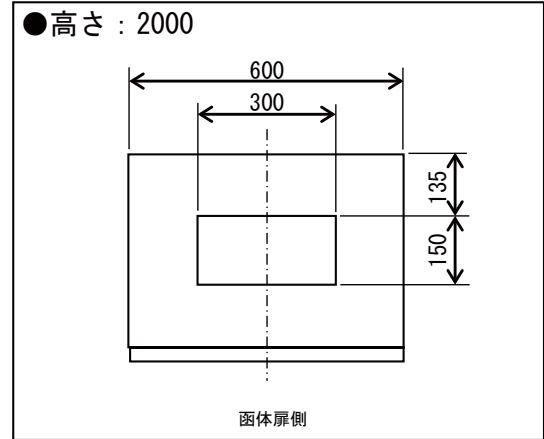
【図3】受信機函体の入線孔寸法図 入線孔は筐体底面にあります。
