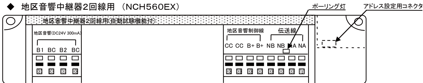
図 : 連結端子
