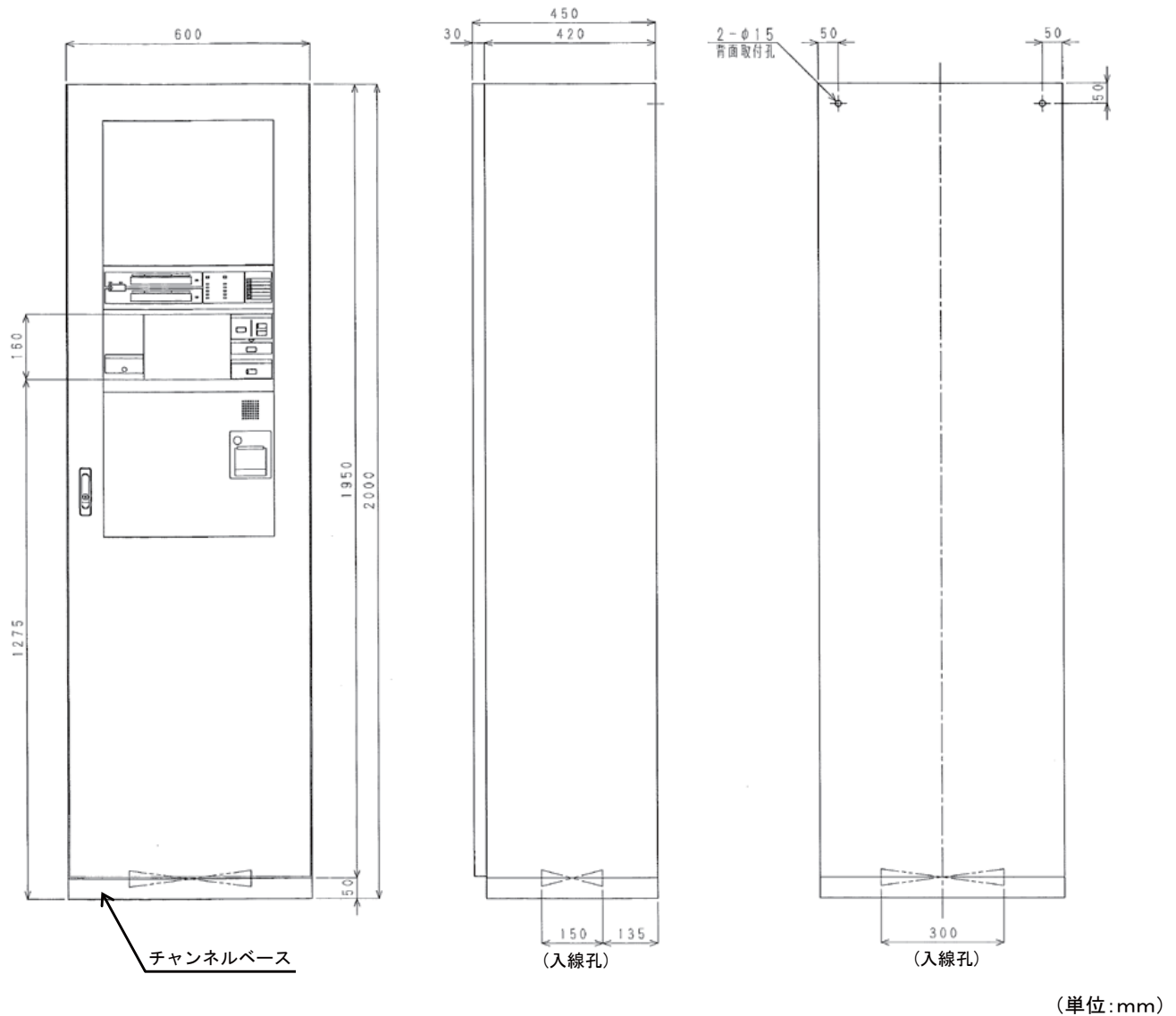
【図1】取付寸法図 (H2000×W600×D450)
