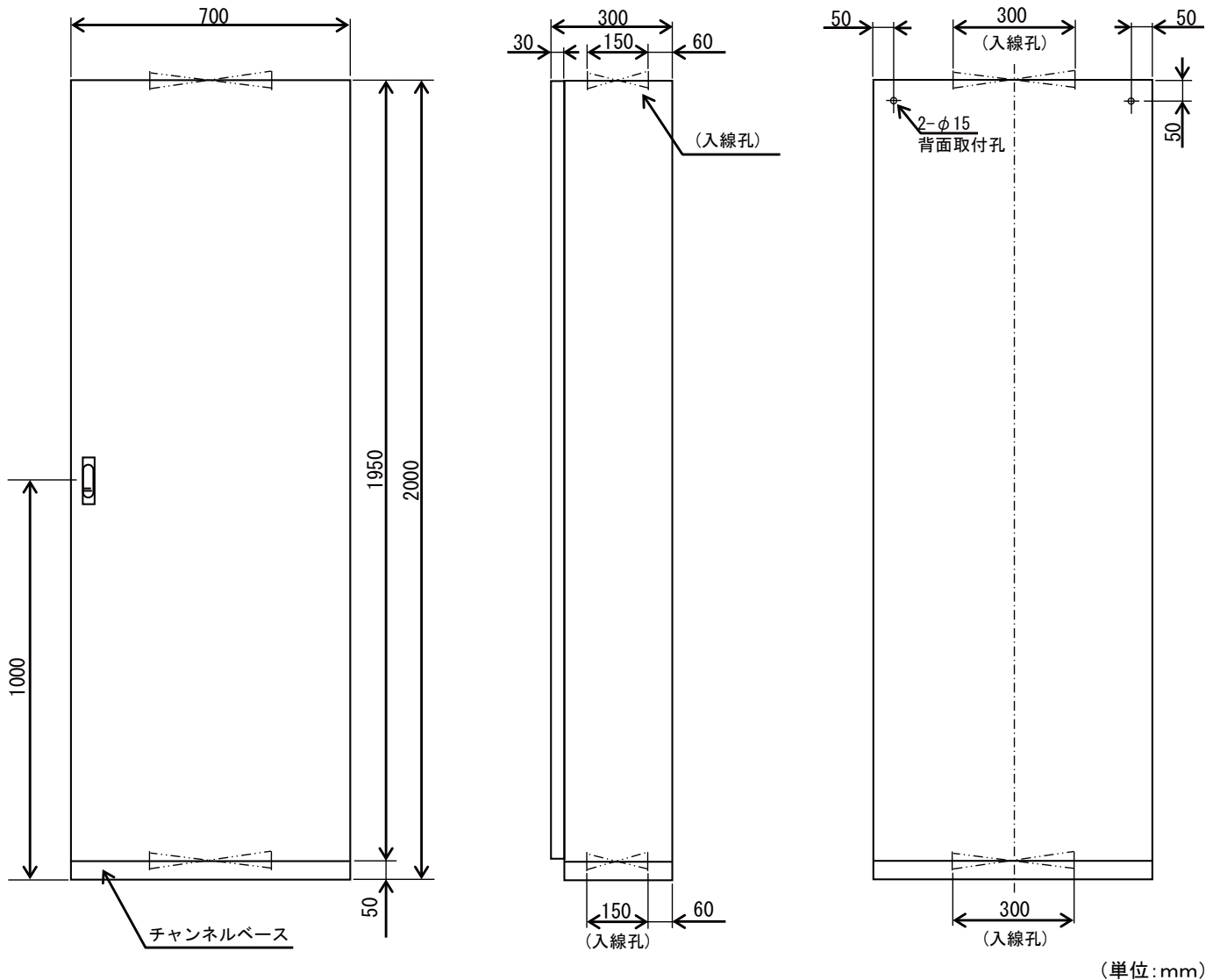
【図4】取付寸法図 (H2000×W700×D300)
