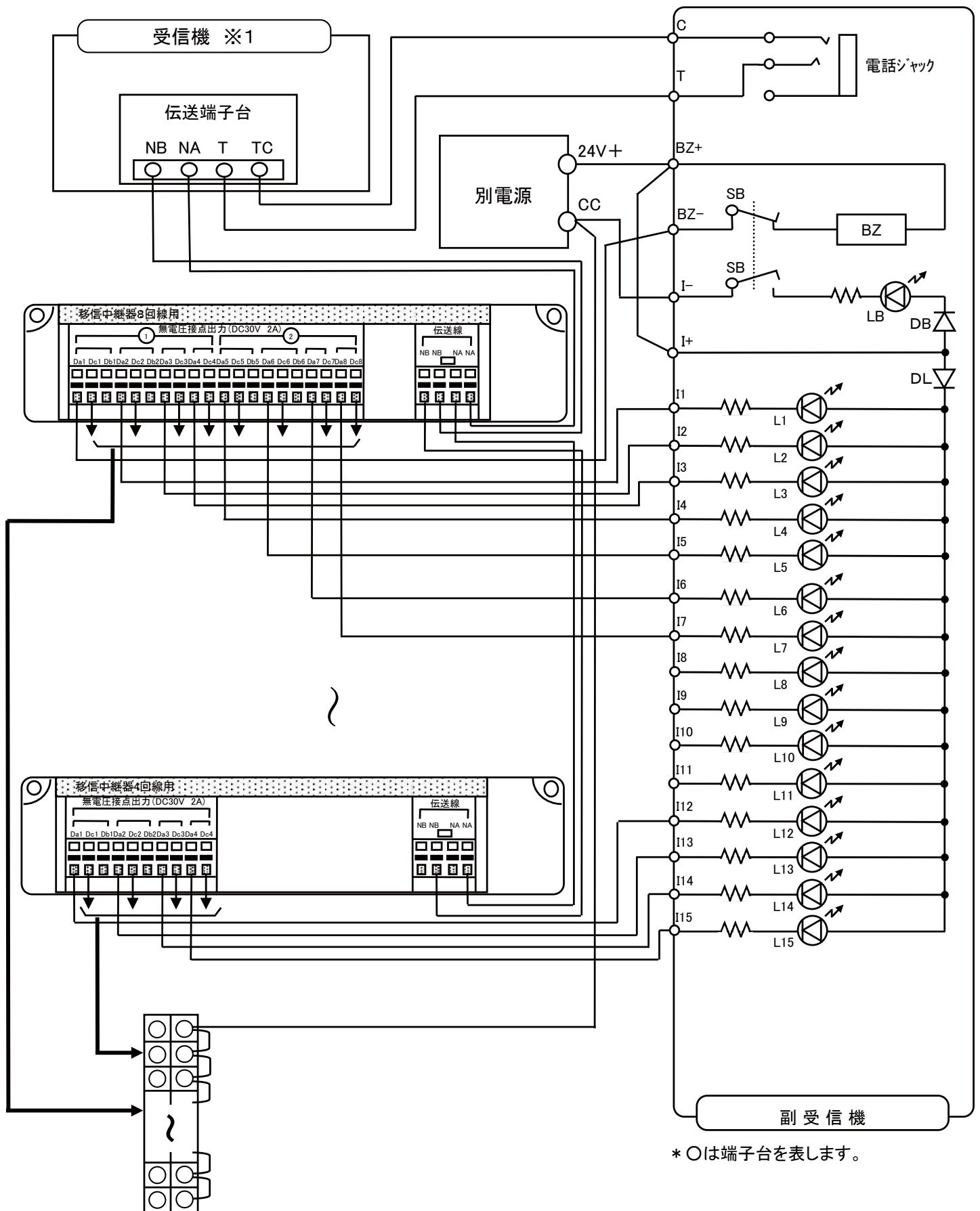
中継端子台
