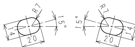
取付用長穴寸法図 (S=1/2)
