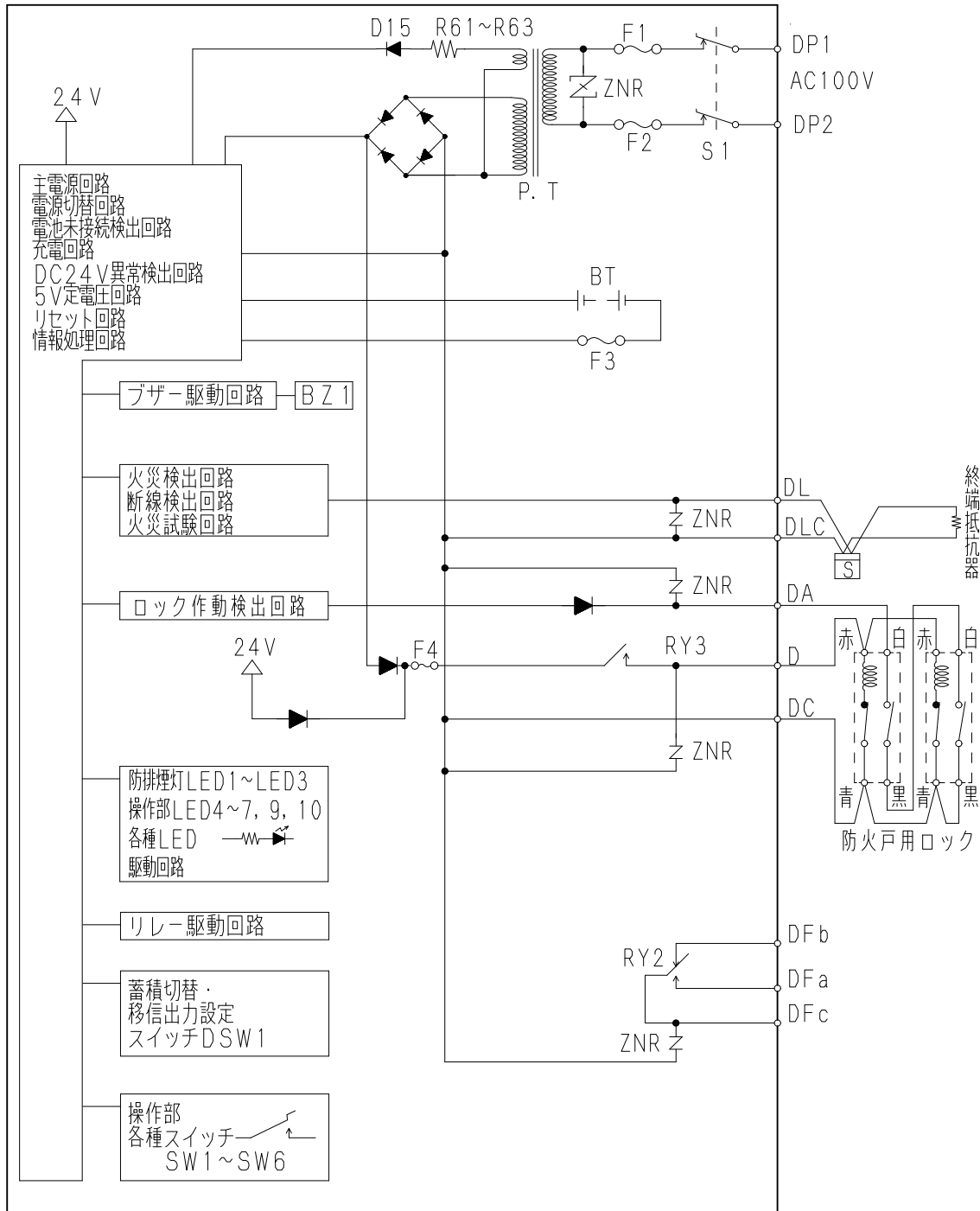
連動制御器
