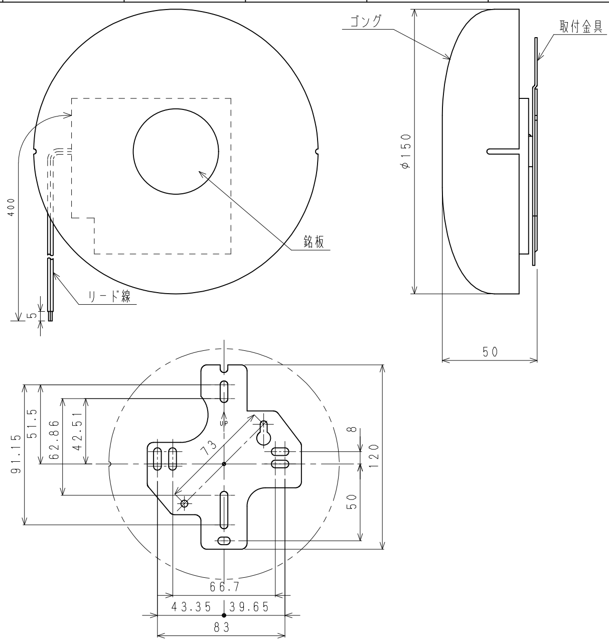
取付板寸法図
