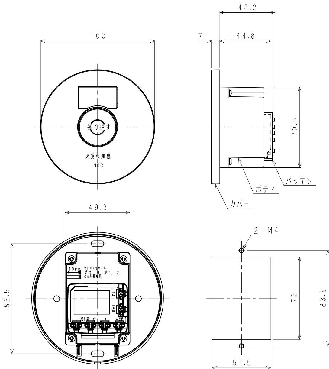
裏面図(端子配置/パッキンなし)
