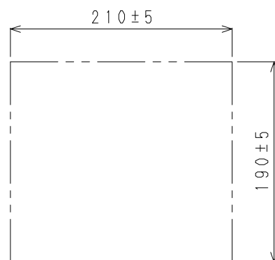
函体埋込穴寸法図
