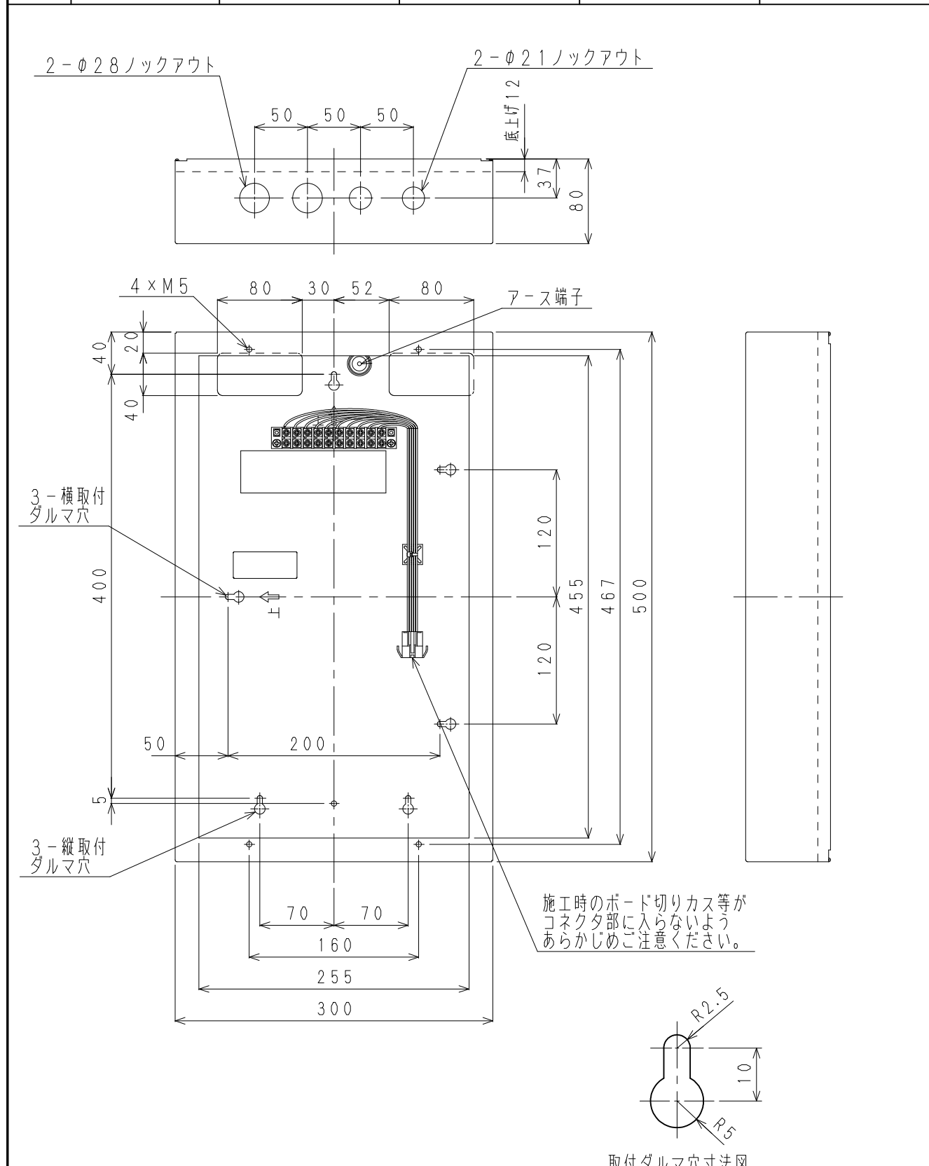
取付ダルマ穴寸法図
