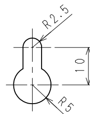
取付ダルマ穴寸法図
