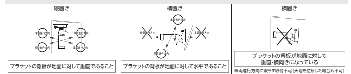
クイックスブラッシャートリガーM・ブラケット取付向きと車両進行方向(○取付可能 ×取付禁止)
