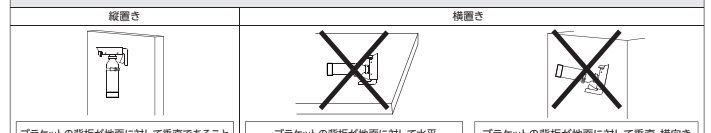
クイックスブラッシャートリガーL・ブラケット取付向き
